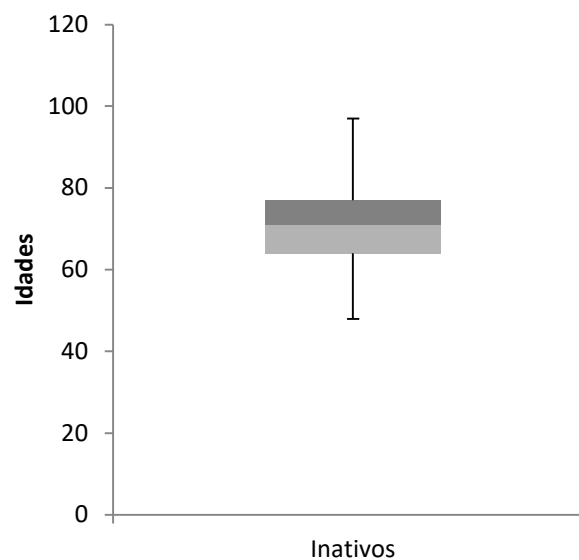
BOXPLOT INATIVOS
